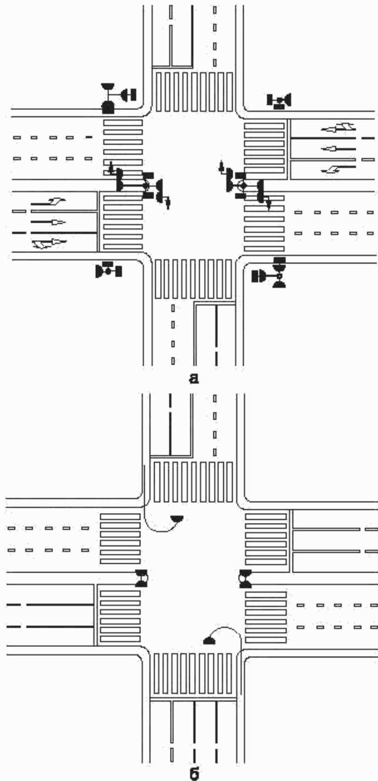
Рисунок В.24 — Пример размещения светофоров: а — на перекрестке; б — на разделительной полосе и над проезжей частью
