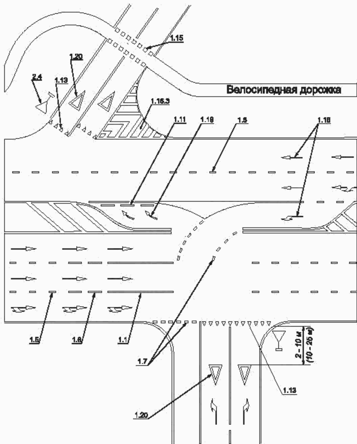
Рисунок В.10 — Пример нанесения разметки канализированного пересечения
